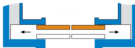
2-paneelinen, keskeltä aukeava
