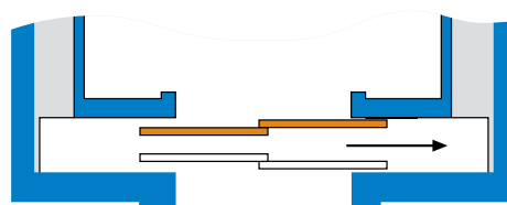
2-paneelinen, sivulle aukeava
