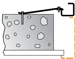
Kapea karmi (LAF1)
