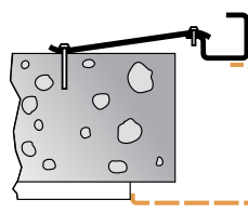
Kapea karmi (LAF2)
