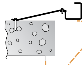
Kapea karmi (LAF3)
