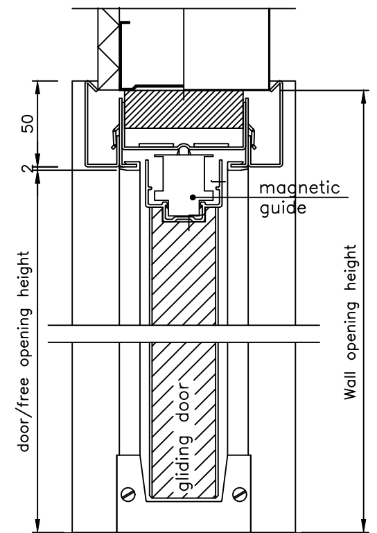
Section C'C
