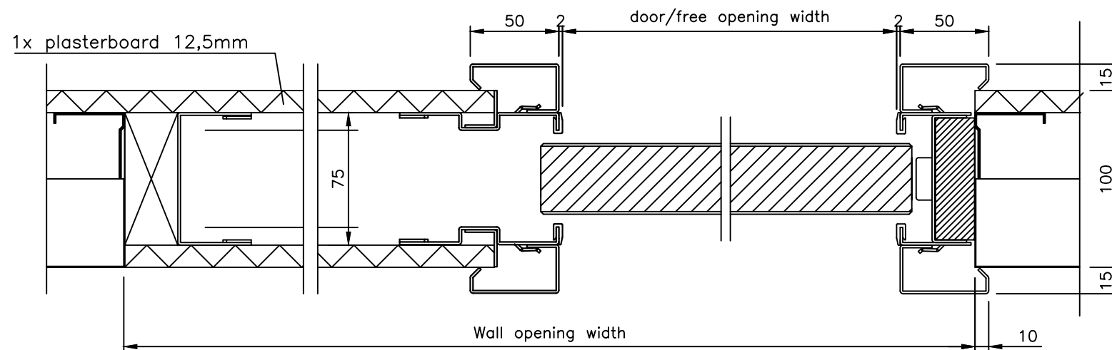
Section A'A
